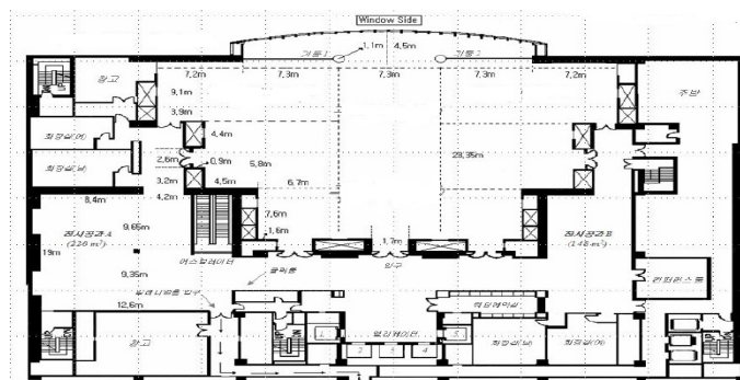
[그림 2-1] 출장 연회 행사장 도면의 예
